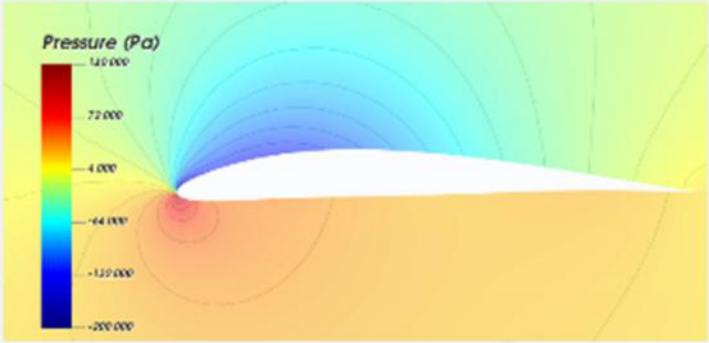
初始翼型
