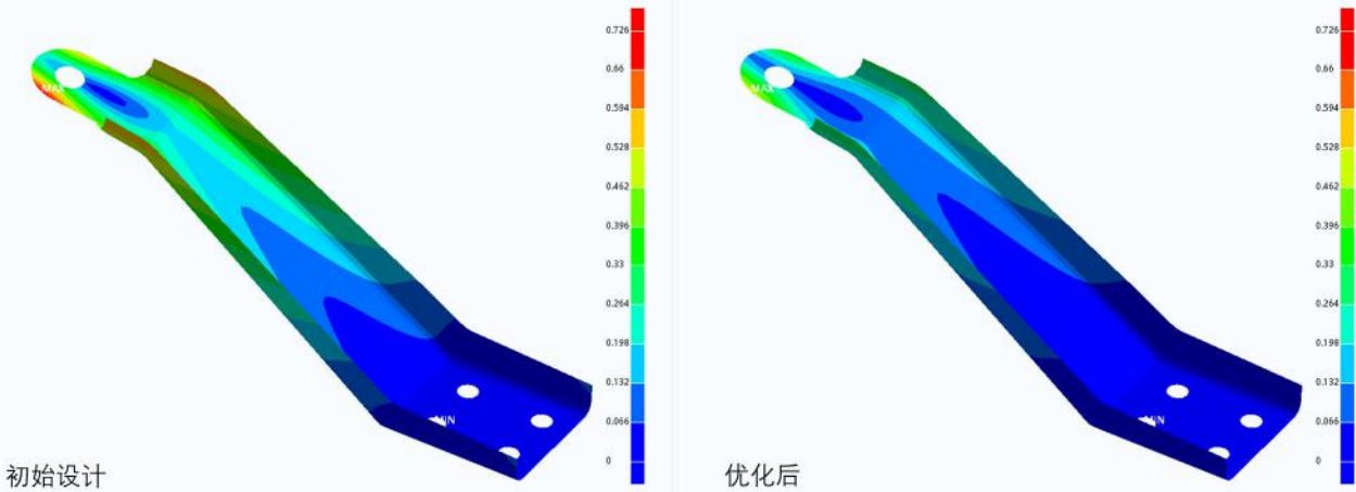
优化前后位移分布
