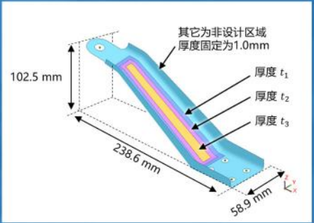
汽车金属板支架示意图
