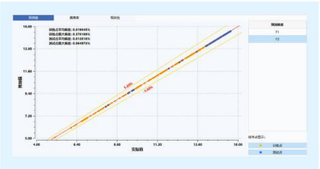
代理模型精度检验--预测结果与实际值对比
