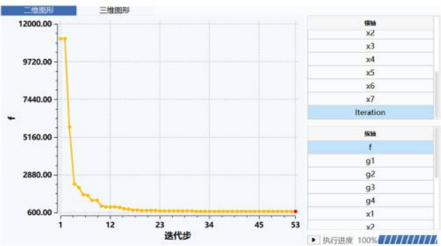
七变量强约束非线性问题优化过程
