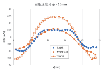
小尺度流化床
