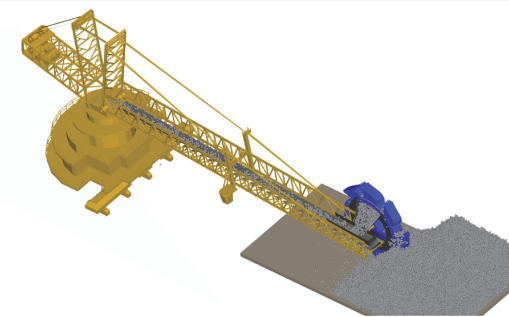
堆取料机
